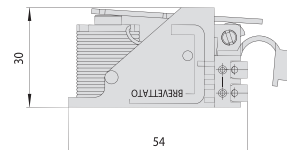
Сменные катушки регулируемые 07.120.00.2 (12V) 07.120.01.2(24V)
