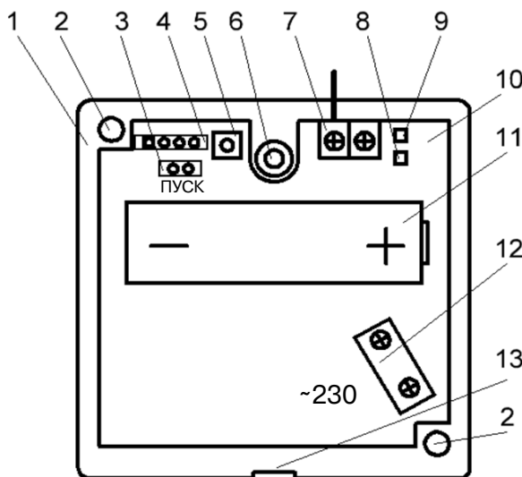
Рисунок 1 – СН-РЕТР со снятой крышкой
